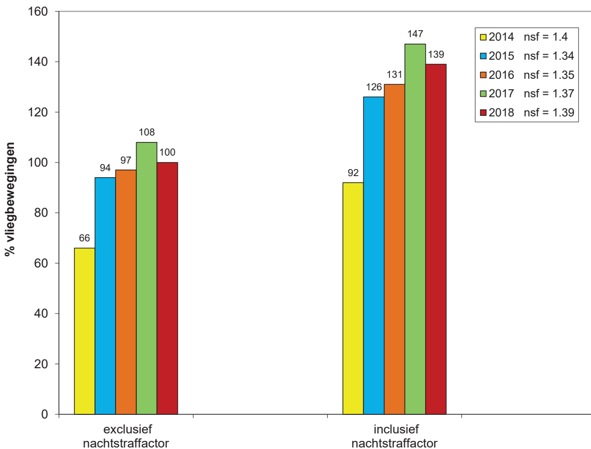
Figuur 1: Percentage vliegtuigbewegingen ten opzichte van het jaar 2018 (exclusief nachtstraffactor = 100%), Vliegbasis Gilze-Rijen
