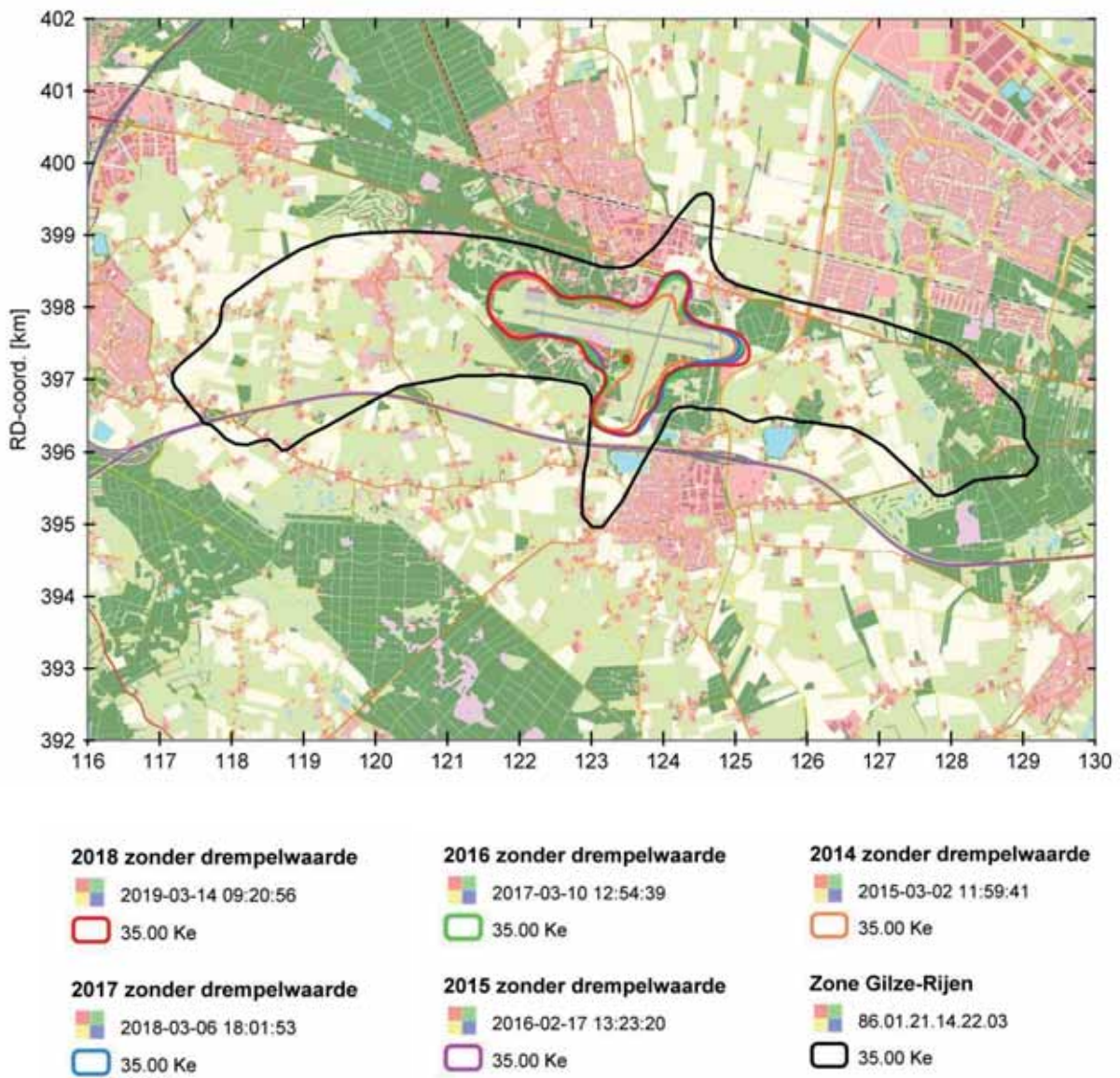
Figuur 4: 35 Ke-geluidbelastingscontouren voor de jaarberekeningen zonder drempelwaarde voor de jaren 2014 tot en met 2018
