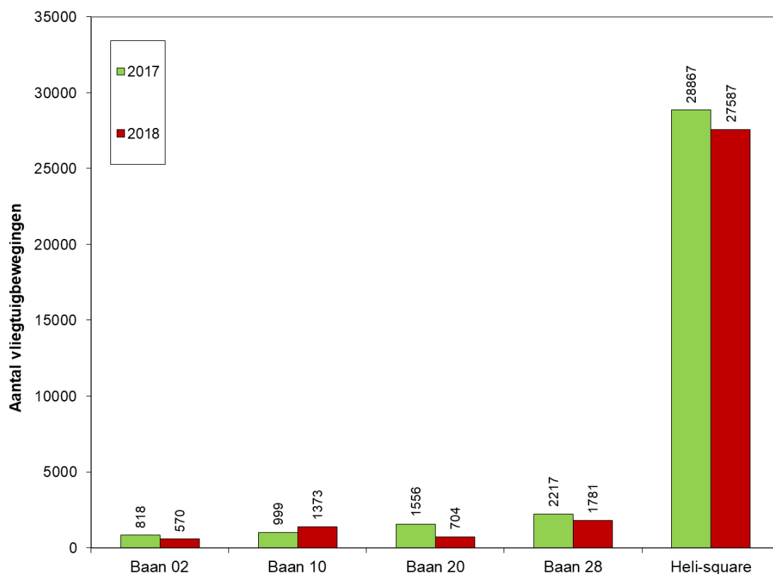
Figuur 1: Aantal vliegtuigbewegingen per baan (exclusief nachtstraffactor), Vliegbasis Gilze-Rijen
