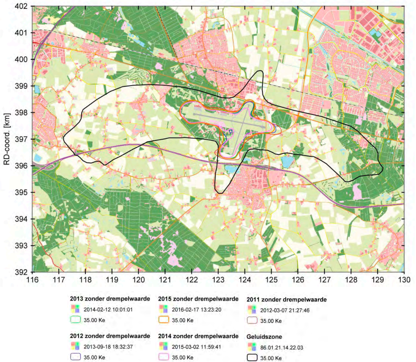
Figuur 4: 35 Ke-geluidbelastingscontouren voor de jaarberekeningen zonder drempelwaarde voor de jaren 2011 tot en met 2015
